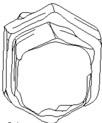
Ruby
