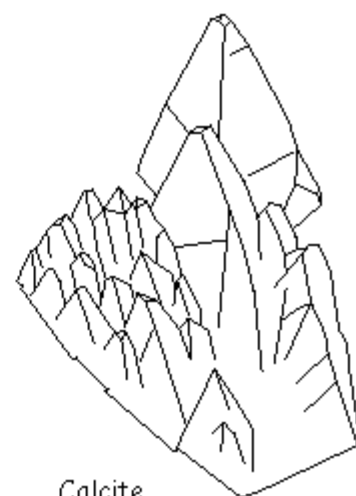
Calcite
