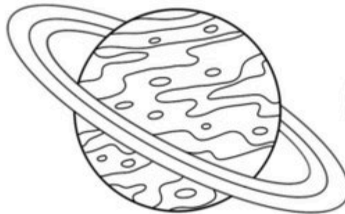
uranus
