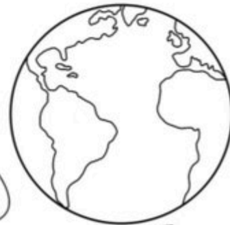
earth
