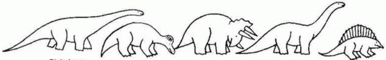
Corythosaurus
