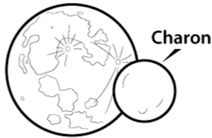
Pluto
