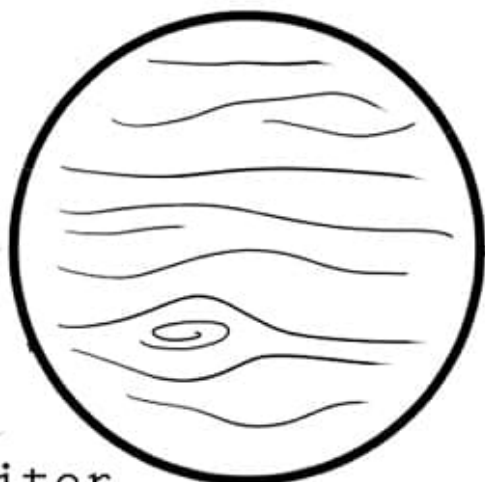
Jupiter
