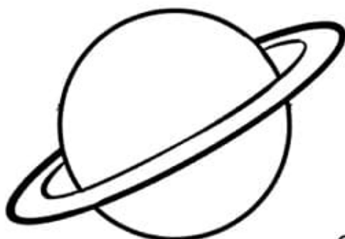
Uranus
